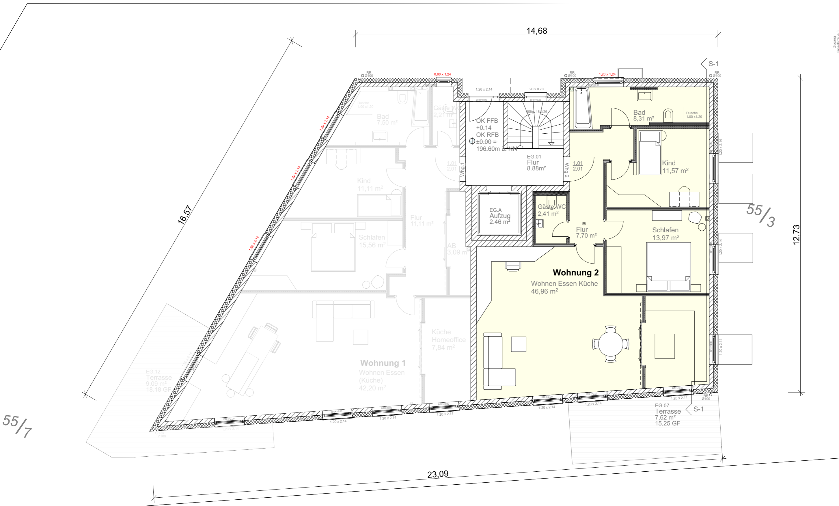
Neubau 6 Familienhaus Kanzelstraße 8, 65191 Wiesbaden Bierstadt Erdgeschoss 1:100 Stand 31.Oktober 2023
